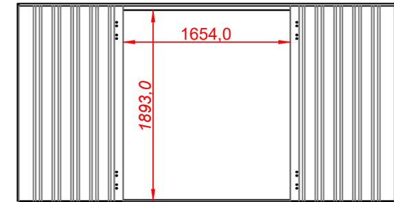
DOUBLE DOOR DIMENSIONS 1893 x 1654 x 35
