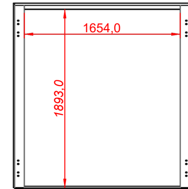
DOUBLE DOOR DIMENSIONS 1893 x 1654 x 35
